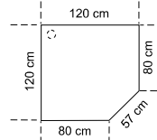
SL-0211 -x xxx xx Spojovací úhel 90° 120 x 120 x 75 cm, 1x opěrná noha
