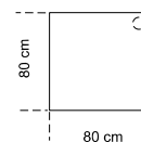
SL-0215 -x xxx xx Spojovací úhel 90° 80 x 80 x 75 cm, 1x opěrná noha
